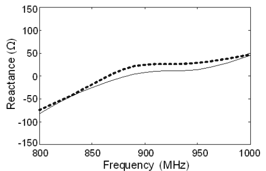
(b) 리액턴스 (b) Reactance
