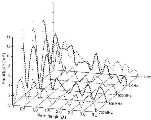
(a) 크기 변화 (a) Amplitude on the strip line
