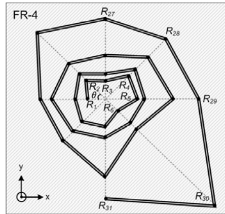
(a) 평면도 (a) Top view
